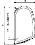
Gehäusemaße (mm)
